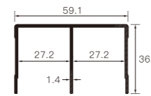
上铝轨道 Upper rail
