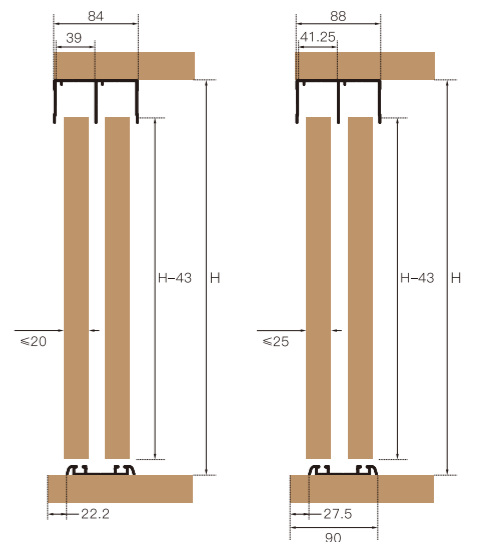
木门 Wood door
