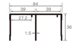
上铝轨道 Upper rail
