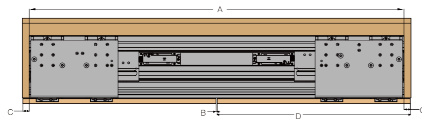
两门柜体参数图 Two doors cabinet parameters
