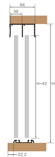
铝框门 Aluminum frame door
