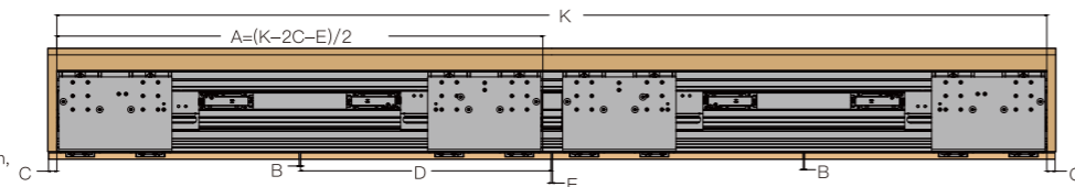
四门柜体参数图 Four doors cabinet parameters
