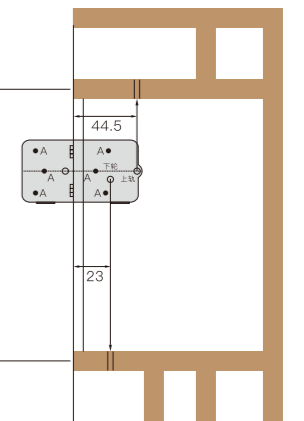
打孔示意图 Drilling Dimension
