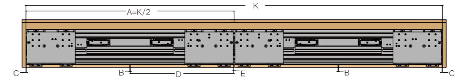
四门柜体参数图 Four doors cabinet parameters
